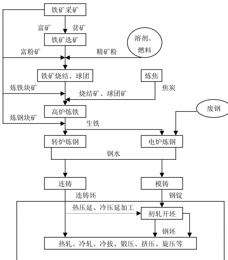
图 B.1 黑色金属冶炼及压延加工项目主要生产流程简图
